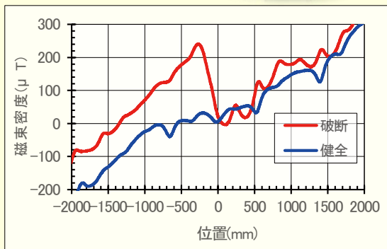
PCポストテンションT桁橋 (鋼製シース、PC鋼線) の実橋調査 測定波形例
